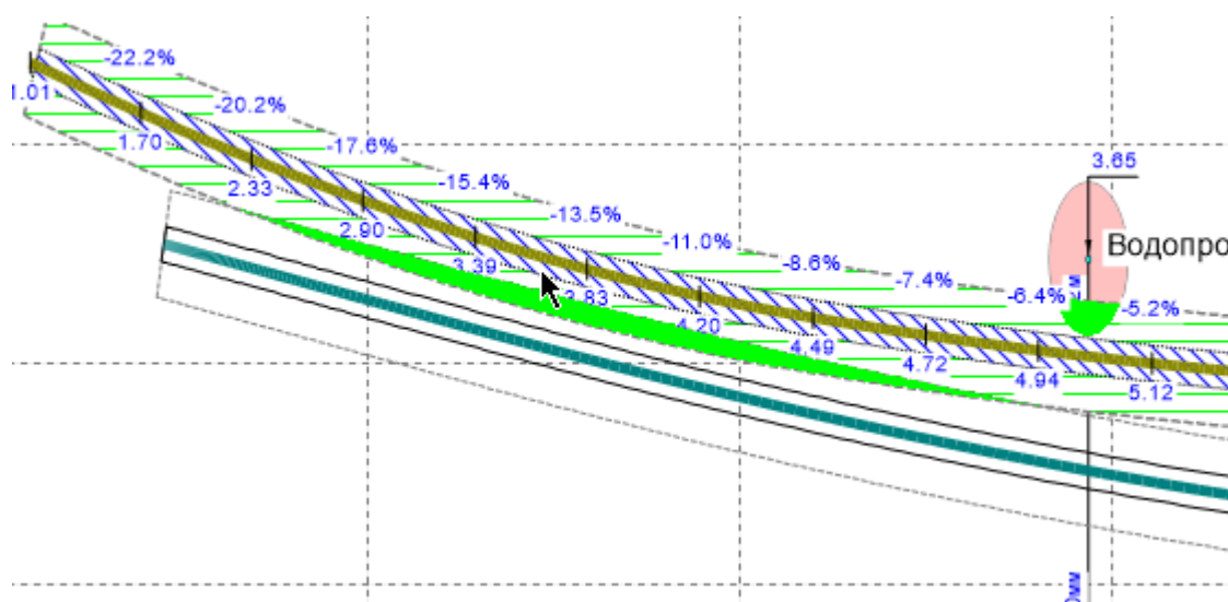
Рис.64 Контрольная зона трассы
