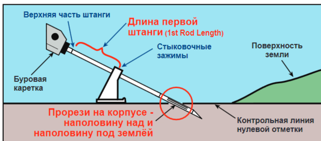
Рис.79 Измерение длины 1-ой штанги
