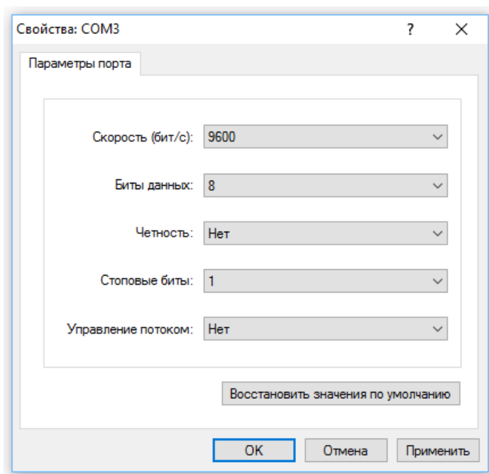
Рис.73 Окно настройки COM порта
