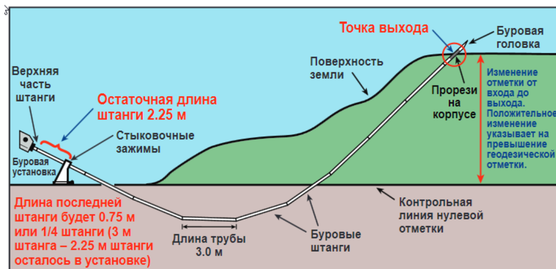
Рис.80 Измерение длины последней штанги
